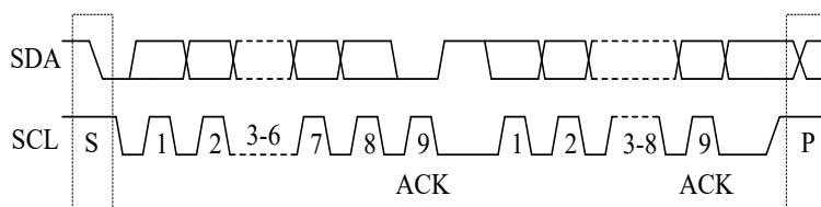
字节格式
