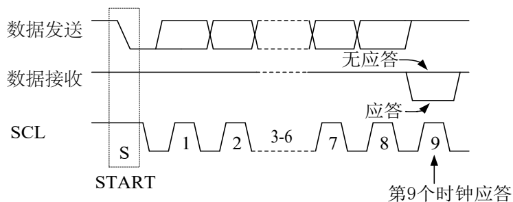
应答信号
