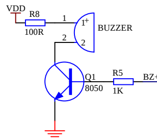
无源蜂鸣器驱动电流>1mA电路
