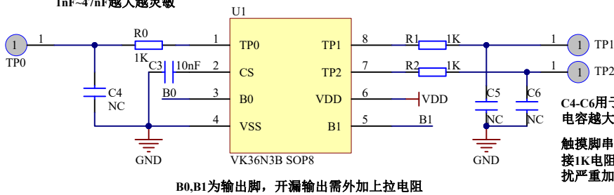
C3用于调节整体灵敏度一般 1nF~47nF越大越灵敏
