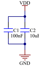
电源脚加滤波电容稳定电源
