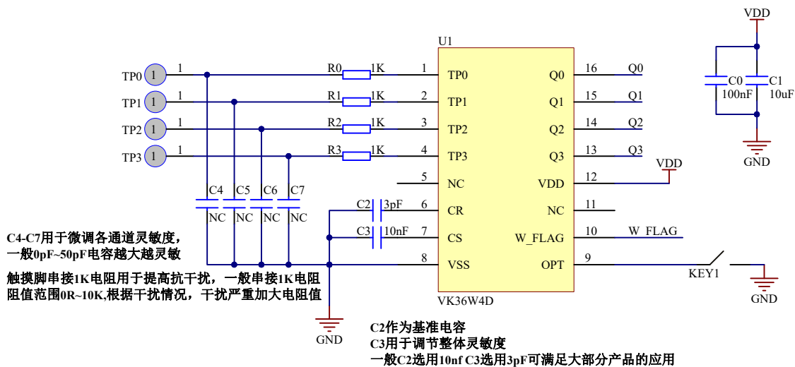
电源脚加滤波电容稳定电源
